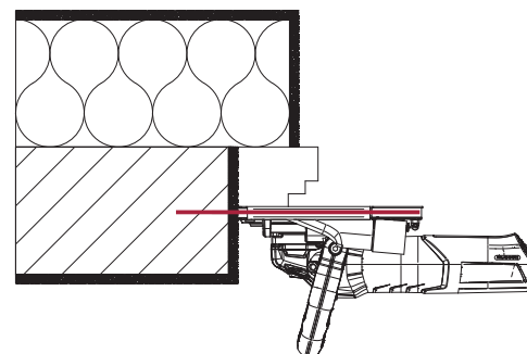
Gerader Schnitt mit 60 mm Tiefe
