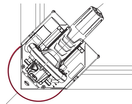
Schnitt bis in die Ecke
