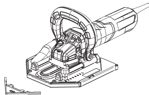
Bodenblech um 180° wenden und Staubschutzzecke aufstecken
