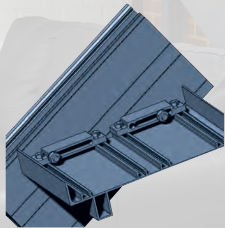
Befestigung der Trittstufen, Befestigung mit Bolzen.
