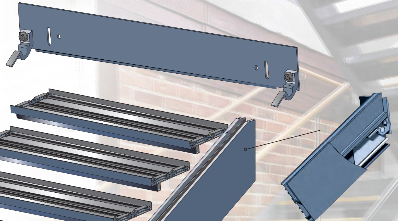
Montage der Anschluss Platte, die Wangen werden an den vorgesehenen Haken der Anschlussplatte befestigt.
